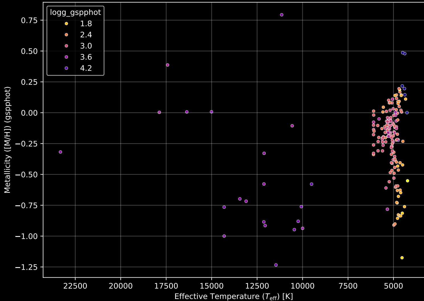
APOGEE DR17 Field: [229-04] Stellar Population Parameters (n= 182)
